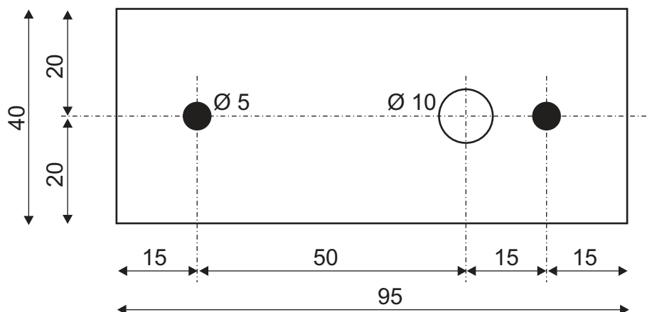
Leuchtenrosette / luminaire canopy
